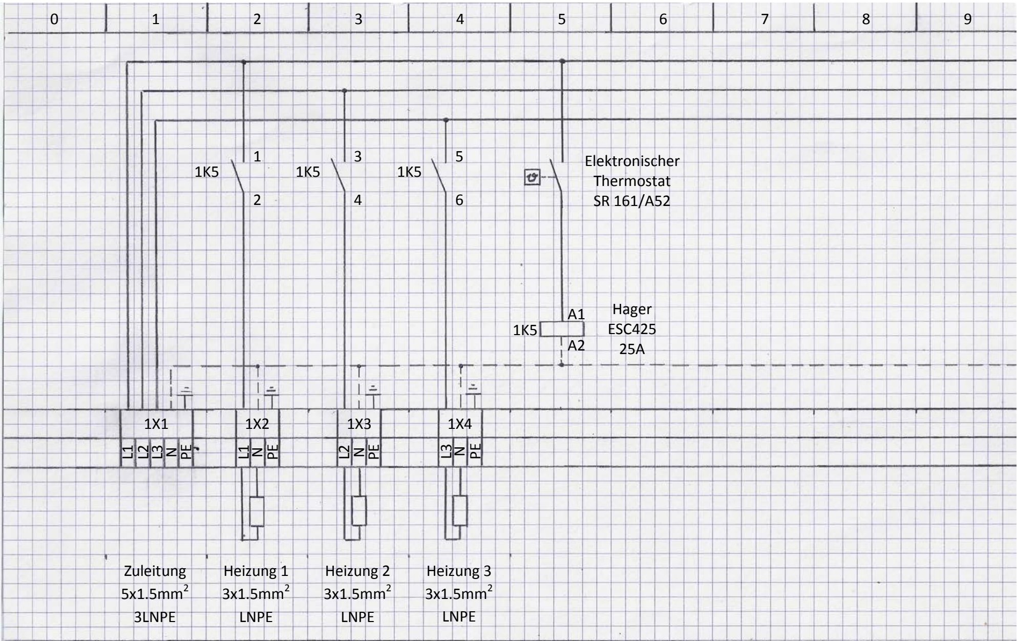
Anschlussschema Maststall Heizung
